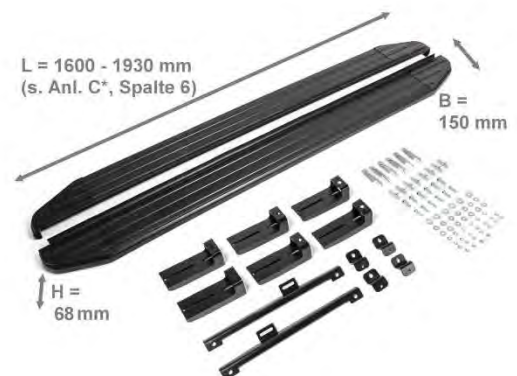
Beispiel für Bausatz (2.A***ALB + Montage- material für Skoda Kodiaq, ab Mj.'17)
